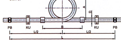
Obr. e. Kompenzační smyčka
